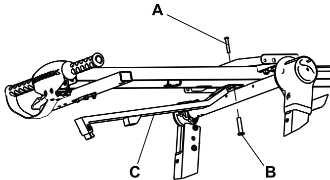
Afbeelding 6 – Haakarm
