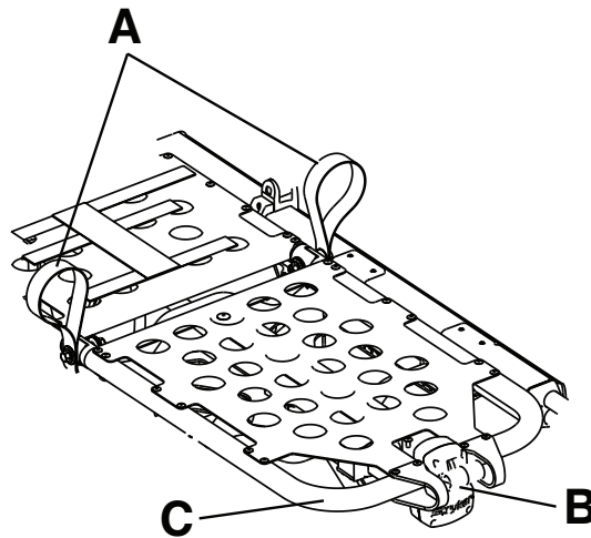
Figur 13 – Knästöd
