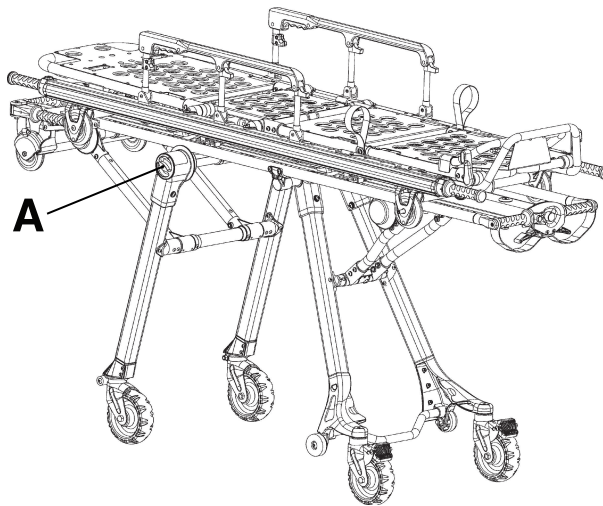
Figura 14 – Posizione del pomello del blocco direzionale
