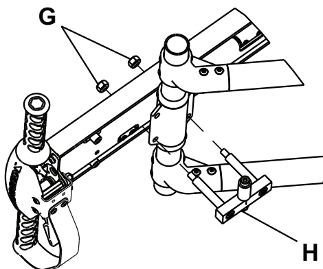
Afbeelding 8 – Rolconstructie
