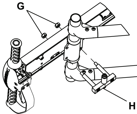
Kuva 8 – Rullakokoonpano
