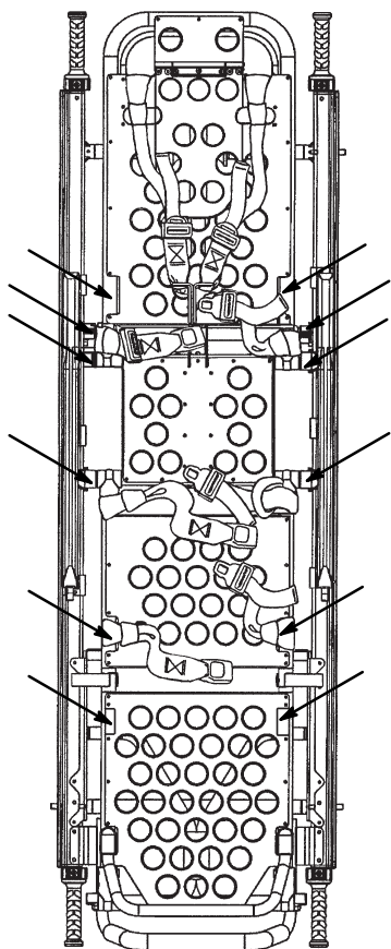
Rysunek 18 – Punkty mocowania pasów unieruchamiających
