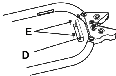
Kuva 11 – Lukituslevy
