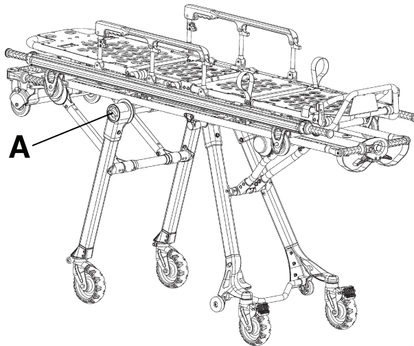
Abbildung 14 – Position des Steer-Lock-Knopfs
