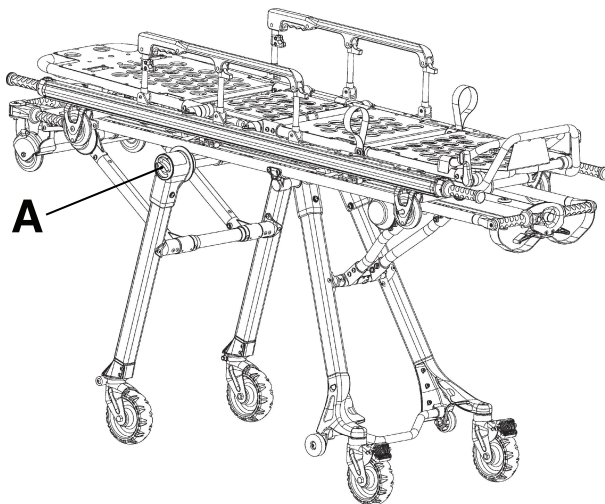
Rysunek 14 – Położenie pokrętła blokady kierunkowych kółek samonastawnych
