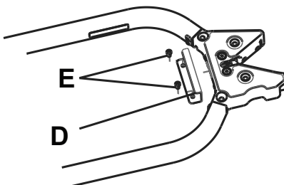
Joonis 11 – Püüdeplaat
