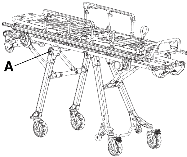
Σχήμα 14 – Θέση περιστρεφόμενου κουμπιού Steer-Lock
