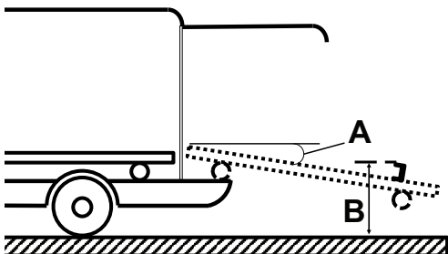
Figur 9 – Spesifikasjoner for bunnplate og lastebrett
