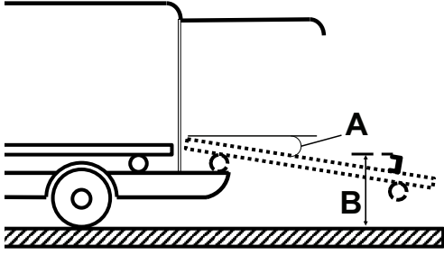
Şekil 9 – Yakalama plakası ve yükleme tepsisi spesifikasyonları
