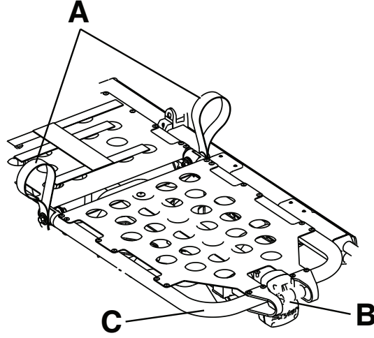
Şekil 13 – Diz bükme desteği
