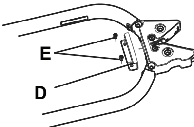
Obrázek 11 – Záchytná deska
