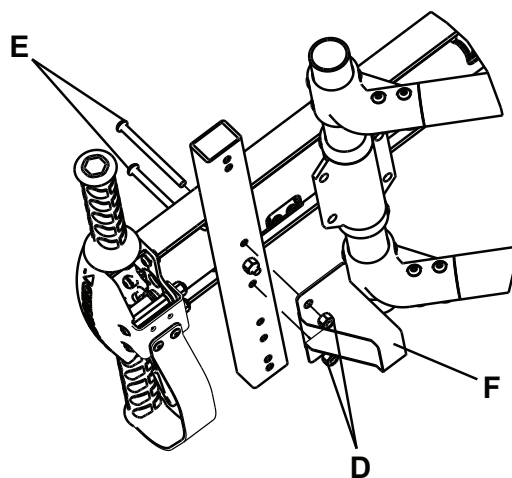
Slika 7 – Vodilo
