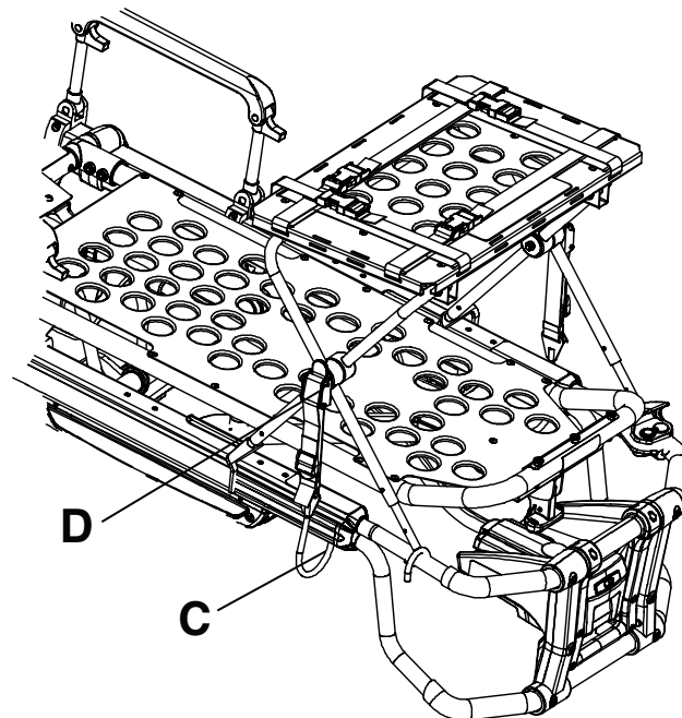
Afbeelding 27 – Plaatsing borghaak (model 6506 weergegeven)
