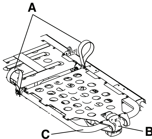
Afbeelding 13 – Knieknikgedeelte
