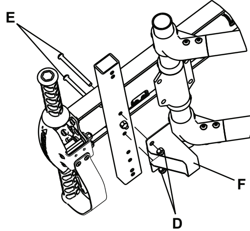
Şekil 7 – Kılavuz braket
